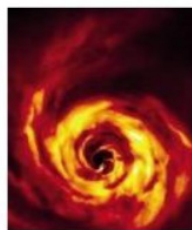
Immagine della nascita di un pianeta in una spirale di gas e polveri, intorno alla stella AB Aurigae ESO, BOCCALETTI
